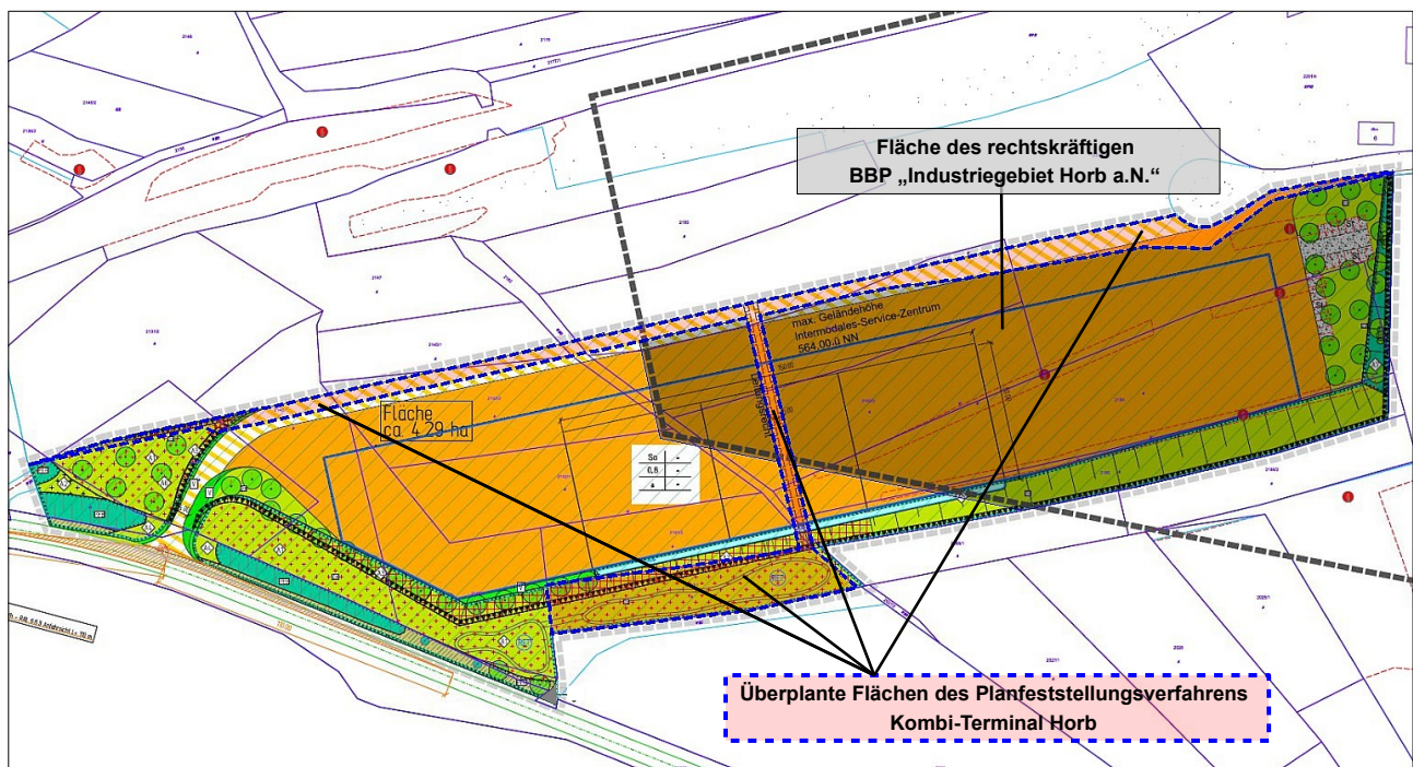
Ausschnitt Bebauungsplan
